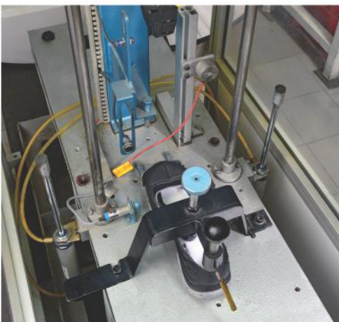
دستگاه آزمون سرپنجه Toe cap test machine
